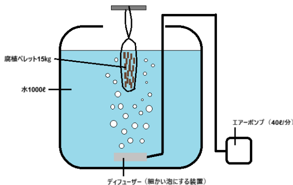
▲ 腐植活性水セットの設置イメージ
